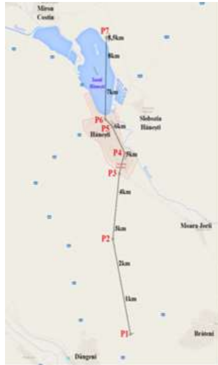
Fig. 14. Tornado trajectory over Hănești, Botoșani County on 11.07.2014 (Pancu, 2014)
